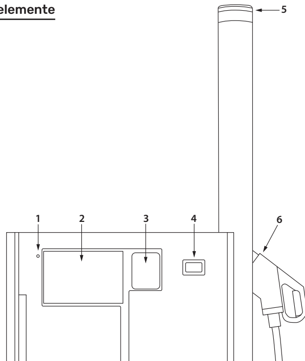
Außenansicht von vorne
