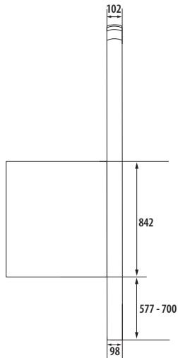
Ansicht von vorne
