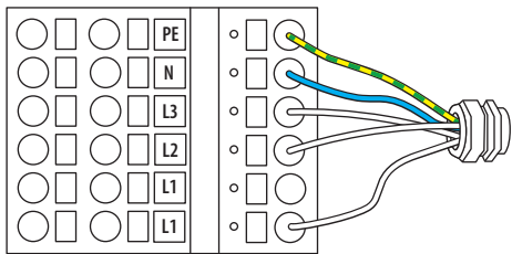
Ansicht bei geöffneter Tür der DC-Wallbox
