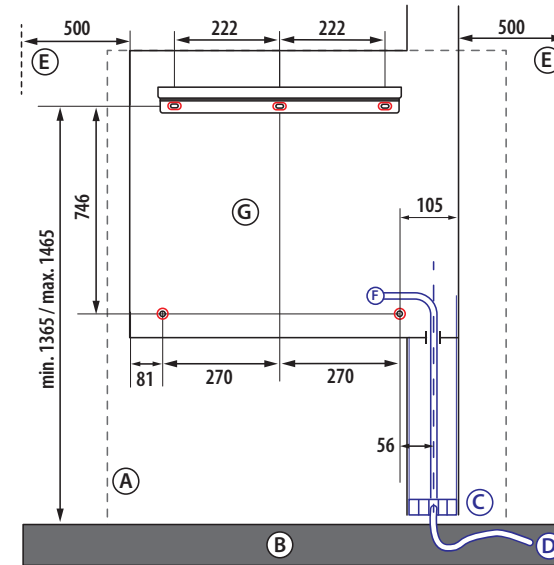
Ansicht auf Montagefläche und Montageschiene
