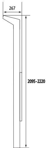
Ansicht von rechts
